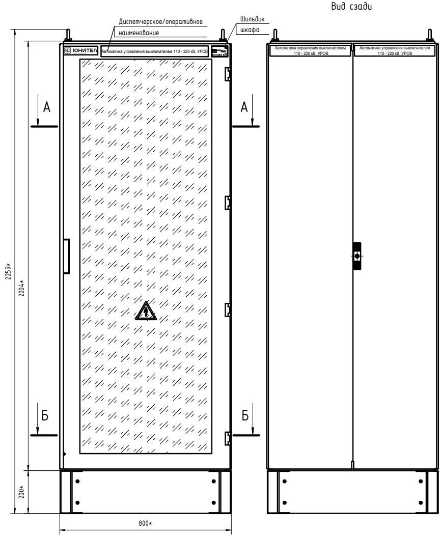
Рисунок Д.1 – Чертеж общего вида
